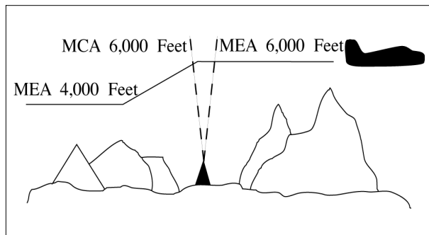
FIG 4-5-2 MCA Specified
